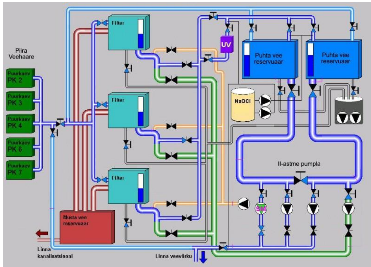
Joonis 5.2. Piira veetöötlusjaama ja II-astme pumpa põhimõtteline skeem
